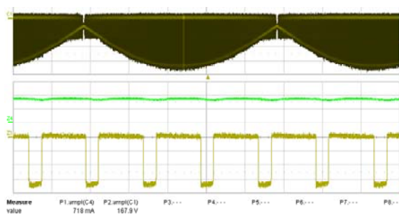
图22 – 265 VAC, 满载
