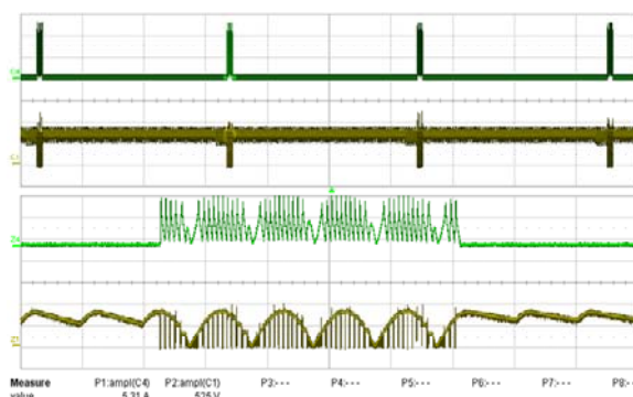
图24 – 265 VAC, 满载
