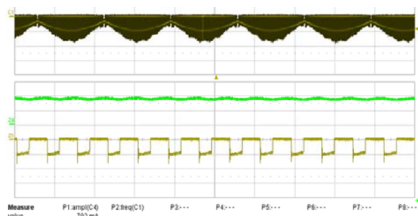
图21 – 110 VAC, 满载
