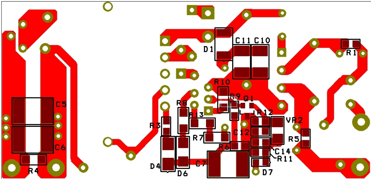
图5 – DER-284板PCB布局, 底视图
