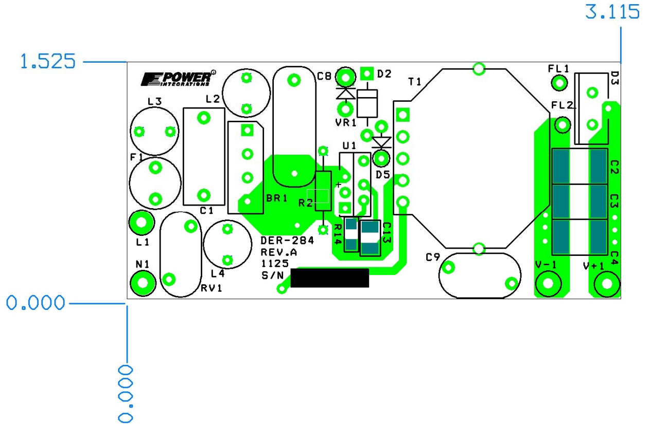
图4 – DER-284板PCB布局，顶视图
