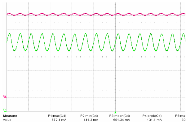
图19 – 265 VAC, 满载。
