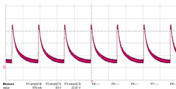
图27 – 输出电压: 230 VAC。 V_{OUT} , 20 V/格, 1 s/格
